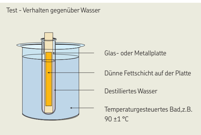
Ölabscheidungstest
