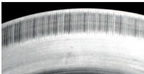
Typische Riffelung bei Funkenerosion in Wälzlagern
